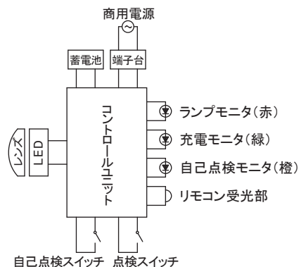
接続図
